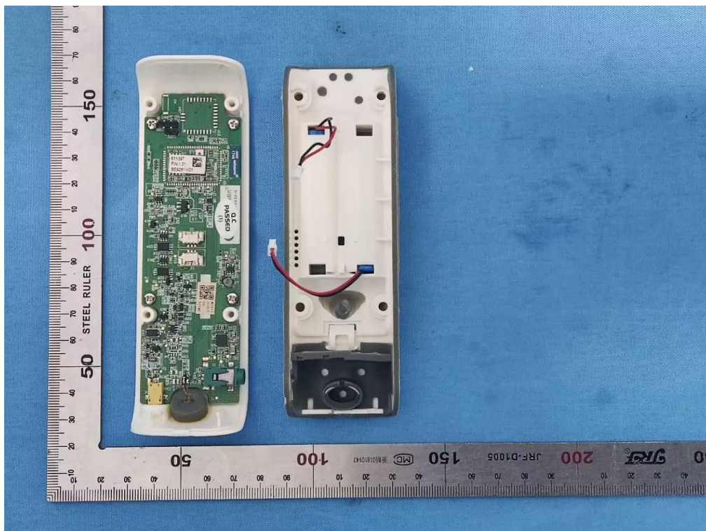
图 6 – 拆机照 (个人交流系统 型号: BE2021)
