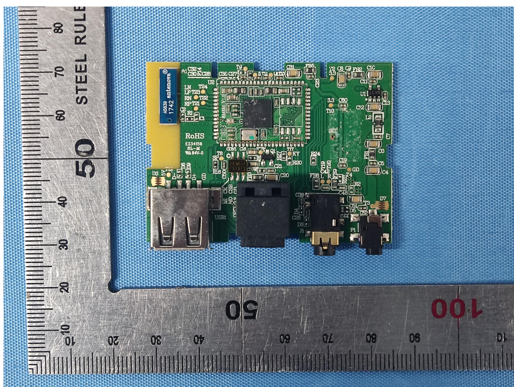
图 14 – 内部照 (电视伴侣 型号: BE2022)
