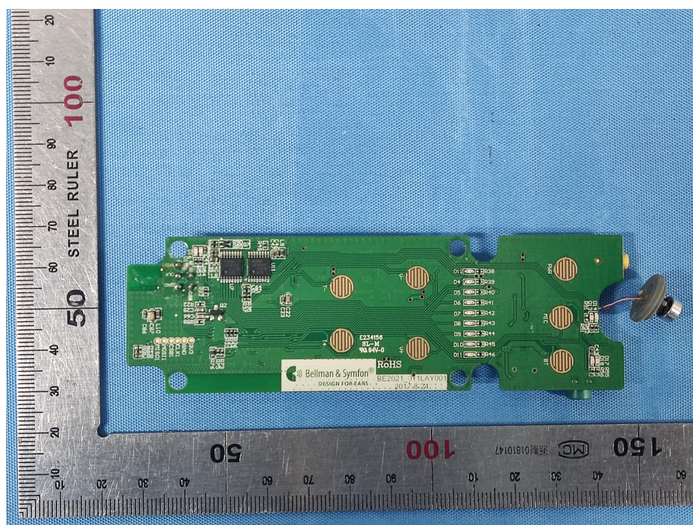
图 8 – 内部照 (个人交流系统 型号: BE2021)
