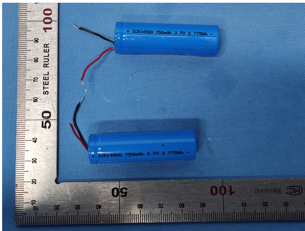
图 9 – 电池照 (个人交流系统 型号: BE2021)
