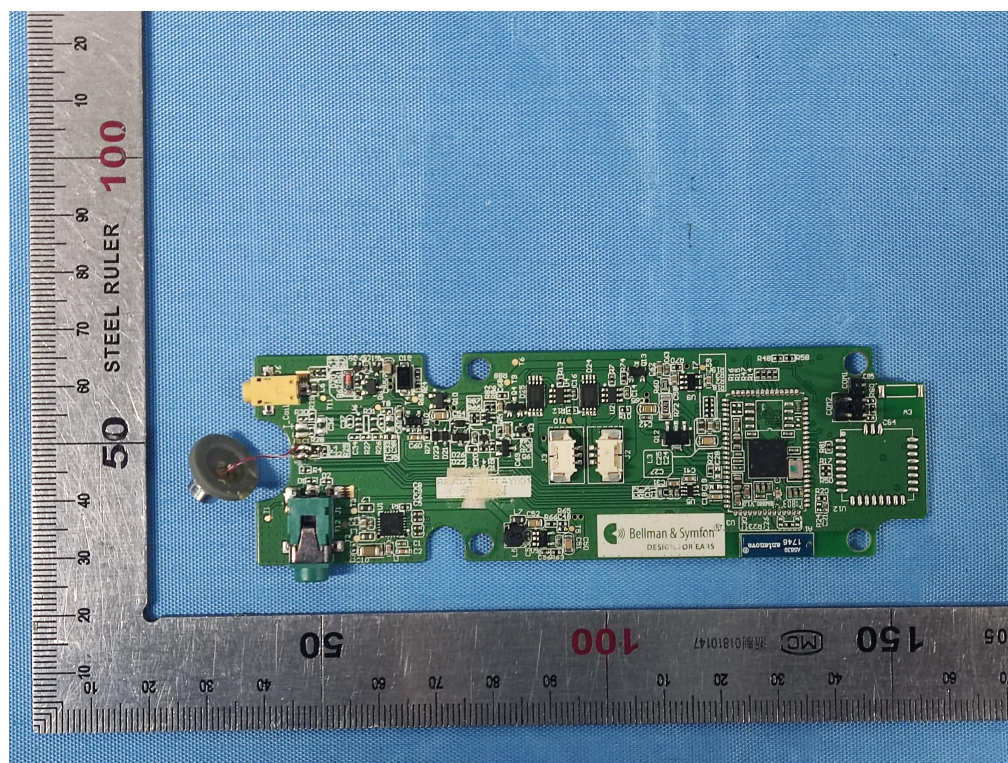
图 7 – 内部照 (个人交流系统 型号: BE2021)
