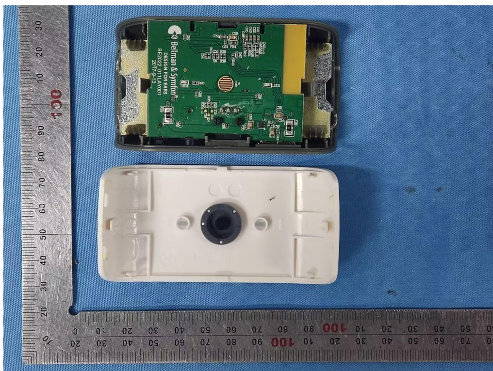
图 13 – 拆机照 (电视伴侣 型号: BE2022)
